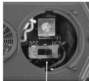
DCC-DCS schalter
